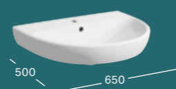
UMIVAONIK, B 650 / T 500 sa otvorom za armaturu, vidljivi preliv bez otvora za armaturu, vidljiv preliv Kompatibiln sa stubom i polstubom
