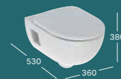
PAKET GEBERIT SELNOVA, B 360 / H 380 / T 530 konzolna WC šolja, vidljivo kačenje, Rimfree® WC sedište sa poklopcem, sporo spuštanje, brza demontaža 501.750.00.1
