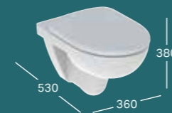
PAKET GEBERIT SELNOVA, B 360 / H 380 / T 530 konzolna WC šolja, vidljivo kačenje, WC sedište sa poklopcem 501.752.00.1
