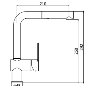
RIN 285CR - RIN 185CR Miscelatore lavello monoforo con doccia estraibile (2 getti) - (RIN185 monogetto) e canna orientabile One-hole sink mixer with pull-out handshower (two-spray) - (RIN185 single-spray) and swivelling spout
