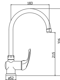
APM3 180CR Miscelatore lavello monoforo con canna tubo orientabile One-hole sink mixer with tube swivelling spout
