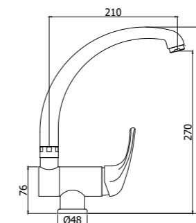
ND 189CR Miscelatore lavello laterale canna reclinabile sotto finestra One-hole sink mixer below window
