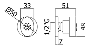
ZSOF 073CR Soffione ellittico in metallo, anticalcare - 48x33 mm Oval metal body jet, antiscald system - 48x33 mm
