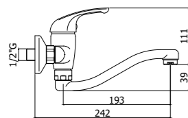
APM3 161CR Miscelatore lavello a muro con canna tubo orientabile Wall sink mixer with swivelling tube spout
