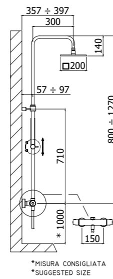
ZCOL 641LIQCR BIRILLO SQUARE Colonna doccia con miscelatore termostatico Shower column with thermostatic mixer
