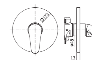
DU BOX010CR Set esterno miscelatore incasso doccia senza deviatore External set for concealed shower mixer without diverter
