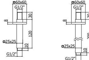
ZSOF 118-119CR Braccio doccia a soffitto - 25x25 mm - L.120/200 mm Ceiling shower arm - 25x25 mm - L.120/200 mm
