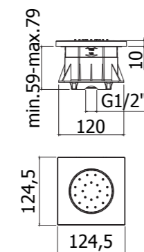
ZSOF 121CR Soffione quadro in ABS, anticalcare, con getto orientabile - 124,5x124,5 mm Square ABS body jet, antiscald system, with swivelling spray - 124,5x124,5 mm
