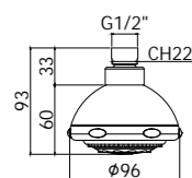
ZSOF 030CR ISCHIA Soffione "Ischia" in ABS, anticalcare Ø 96 mm "Ischia" ABS shower head, antiscald system Ø 96 mm
