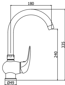
DU 180CR Miscelatore lavello monoforo con canna tubo orientabile One-hole sink mixer with tube swivelling spout
