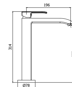
LES 188CR Miscelatore lavello monoforo alto corpo orientabile One-hole tall swivelling sink mixer
