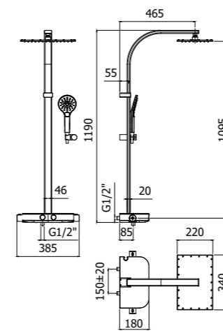
ZCOL 668CR MOBY Colonna doccia con miscelatore termostatico Shower column with thermostatic mixer
