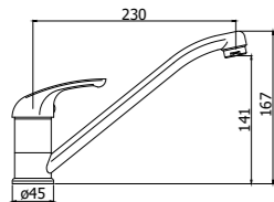
APM3 182CR Miscelatore lavello monoforo con canna tubo orientabile One-hole sink mixer with tube swivelling spout
