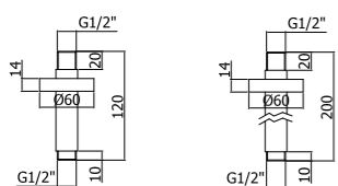
ZSOF 064-065CR Braccio doccia a soffitto - Ø 24 mm - L.120/200 mm Ceiling shower arm - Ø 24 mm - L.120/200 mm
