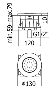
ZSOF 120CR Soffione tondo in ABS, anticalcare, con getto orientabile - Ø130 mm Round ABS body jet, antiscald system, with swivelling spray - Ø130 mm
