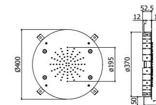
ZSOF 130CR FILADELFIA Soffione ad incasso in metallo, anticalcare, con NEBULIZZATORE - Ø 400 mm Concealed ceiling metal shower head, antiscalc system, with NEBULIZER JETS - Ø 400 mm
