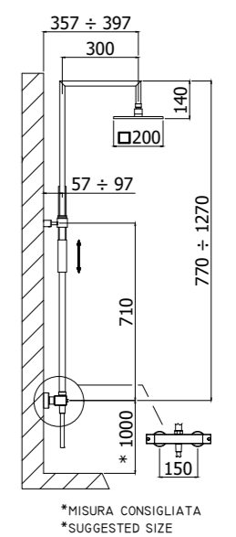
ZCOL 655CR SYNCRO TOP Colonna doccia con miscelatore termostatico Shower column with thermostatic mixer
