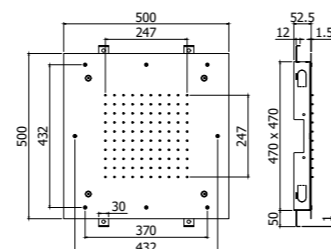
ZSOF 129CR CLEVELAND Soffione ad incasso in metallo, anticalcare, con NEBULIZZATORE - 500x500 mm Concealed ceiling metal shower head, antiscalc system, with NEBULIZER JETS - 500x500 mm
