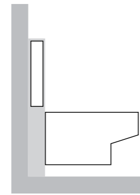
Конзолно решение, предсидна монтажа
